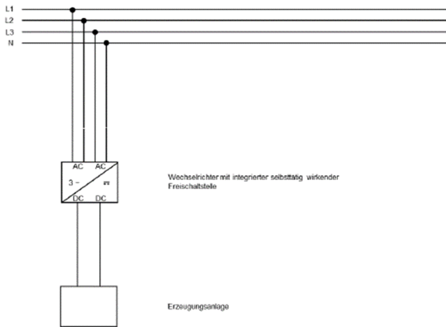
Abbildung 19: Netzanschluss bei Einsatz einer selbsttätig wirkenden Freischnittstelle für mehrphasige Wechselrichter (max. 30 kVA)
